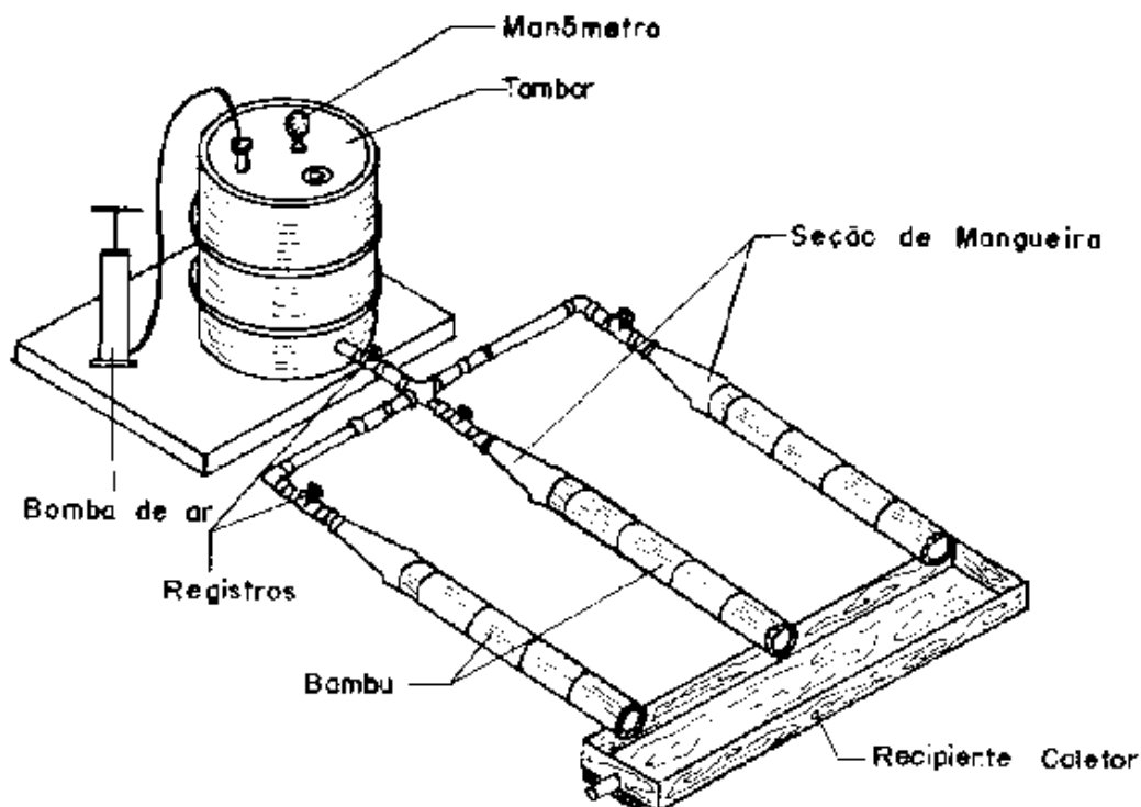
Figura 4. Equipamento para tratamento pelo método boucherie.
