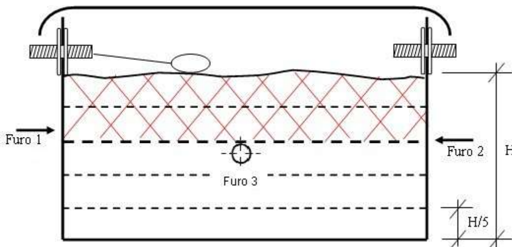
Figura 3 - Posição dos furos no reservatório térmico misto
