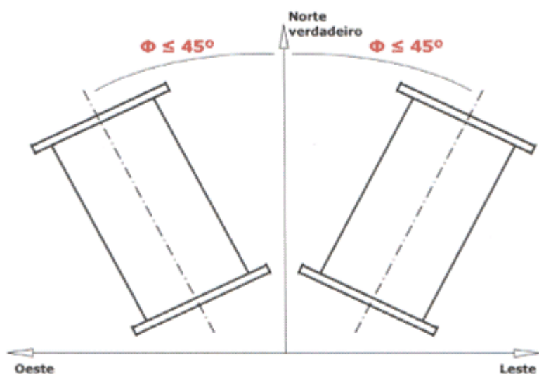
Figura 01: Direção de uma das águas do telhado
